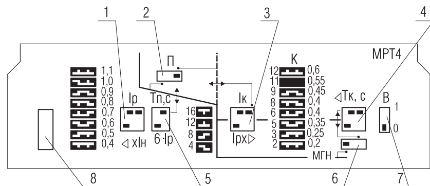
Рисунок 2 - Расцепитель электромагнитный
