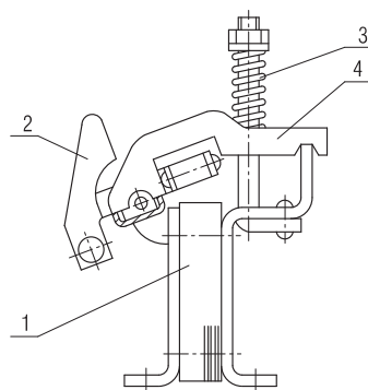
1 - сердечник, 2 - якорь, 3 - пружина, 4 - скоба
