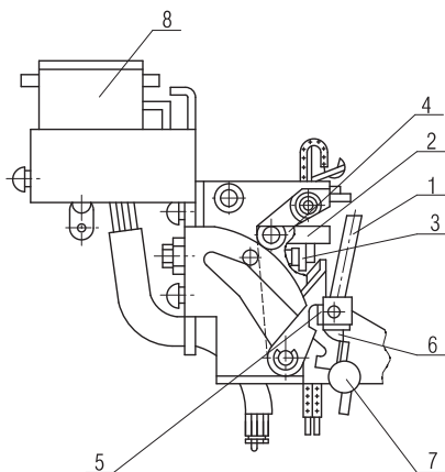
Рисунок 5 - Исполнительный электромагнит МТЗ.
