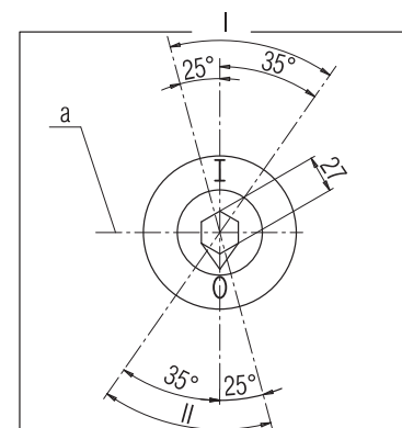
I - зона "Включено"; II - зона "Отключено" a - горизонтальная ось привода.
