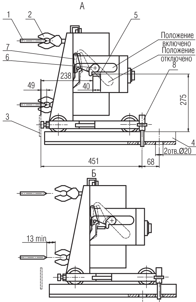
А - рабочее положение, Б - контрольное положение. 1 - шина распределительного устройства (РУ); 2 - врубные контакты выключателя; 3 - упор РУ; 4 - рельсы РУ; 5 - упор блокировки РУ; 6 - рычаг блокировки выключателя; 7 - рычажный механизм блокировки; 8 - фиксатор выключателя.
