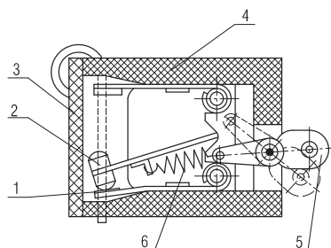
1 - контакт вспомогательный, 2 - контакт подвижный, 3 - крышка, 4 - корпус, 5 - рычаг, 6 - пружина Рисунок 7 - Контакт вспомогательной цепи.
