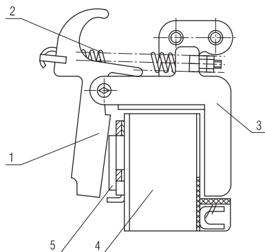
1 - якорь, 2 - пружина, 3 - ярмо, 4 - катушка, 5 - сердечник Рисунок 6 - Расцепитель нулевого напряжения.
