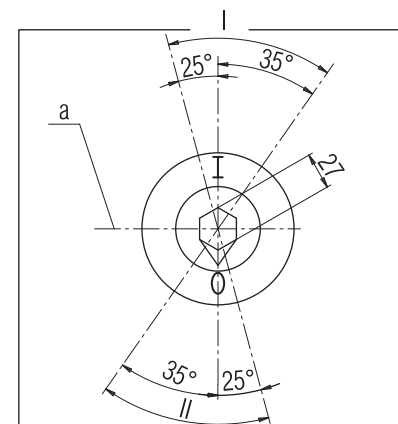
Рисунок 11 - Вкатное устройство выдвжных выключателей.
